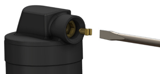
Рис. 10. Демонтаж пробки воздухоотводчика
