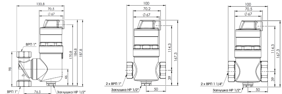
Рис. 2. Размеры сепараторов воздуха (соответственно с левой стороны) AAS 260 / 280 / 281
