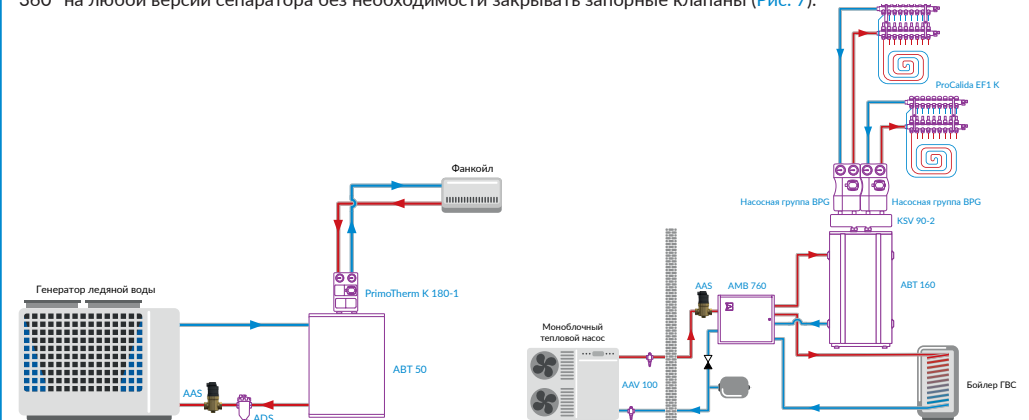
Рис. 3. Примеры систем с сепаратором воздуха AAS
