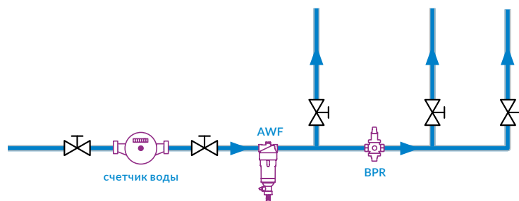
Рис. 2. Примерная схема применения редуктора BPR в системе
