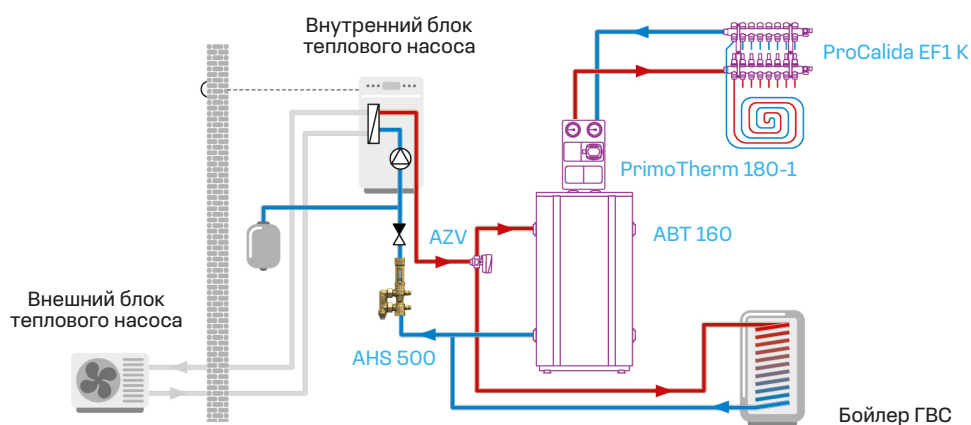
Схема системы с комплектом сервисной арматуры для тепловых насосов AHS 500
