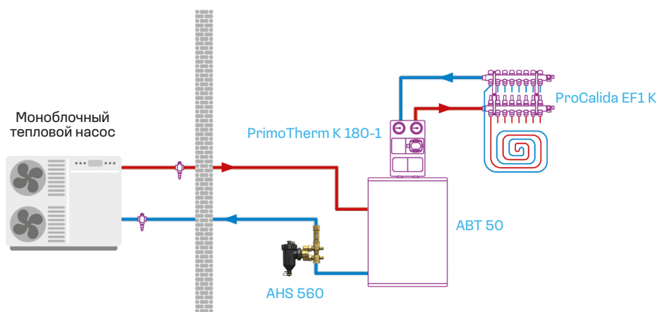
Схема системы с комплектом сервисной арматуры для тепловых насосов AHS 560
