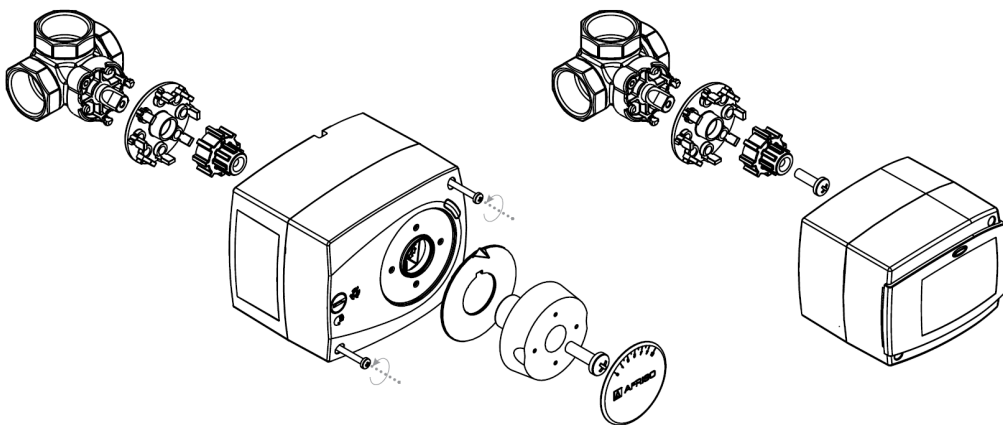
Рис. 2. Монтаж привода ARM/регулятора ACT
