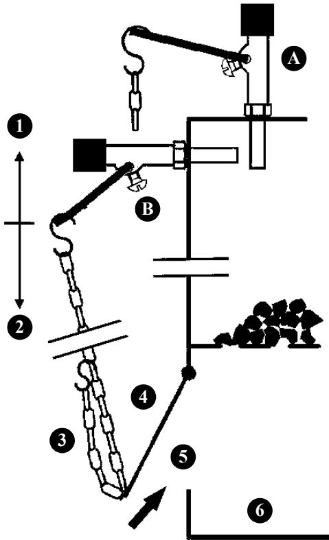
Рисунок 1: Монтажное положение
